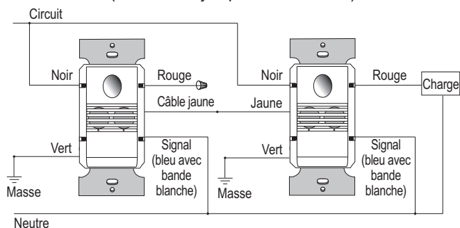
Câblage biphasé
