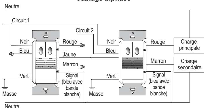
Câblage biphasé
