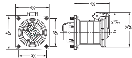
Receptacle
