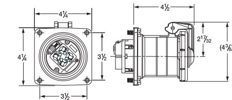
Receptacle
